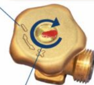
kierunek ZAMYKANIA zaworu butli
